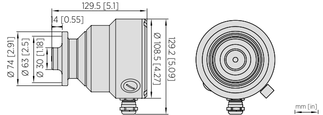
Dimensions PR53GC
